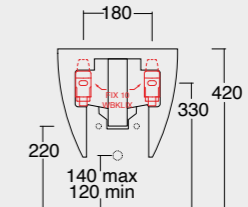
Cod. 45010101 Bidet sospeso Wunder Wunder bidet wall hung
